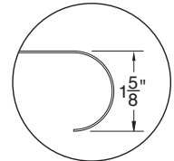
Bull Nose Edge Detail
