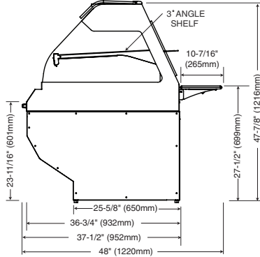
ED2SYS-48/2S Profile
