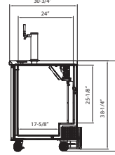
SIDE NLDD24
