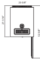
TOP NLDD24
