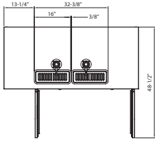
TOP NLDD59
